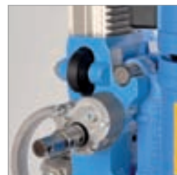
Ansträngningsfritt, ergonomiskt arbetssätt tack vare finmatningsväxeln ( i = 1:3,5 )
